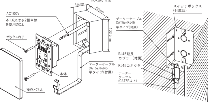
図4. 壁に埋め込み時の施工
