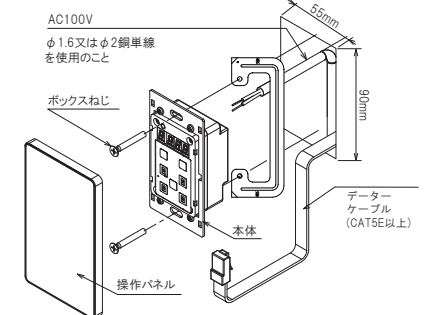
図7. 施工図
